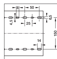
Dno kanala po EN 50085 širina kanala 200 mm
