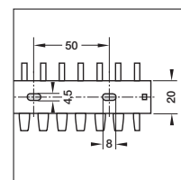
Lajsna za pričvršćivanje VK flex 40
