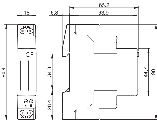
Type 7E.64.8.230.0001
