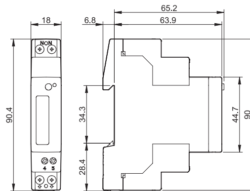
Type 7E.64.8.230.0010
