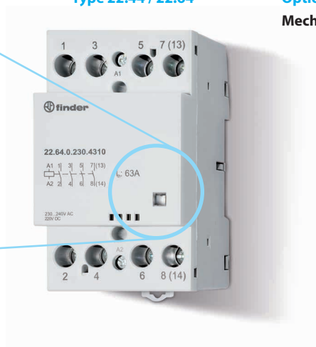
Type 22.44 / 22.64
